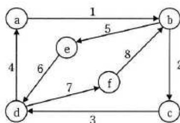
図1 強連結な有向グラフの例
