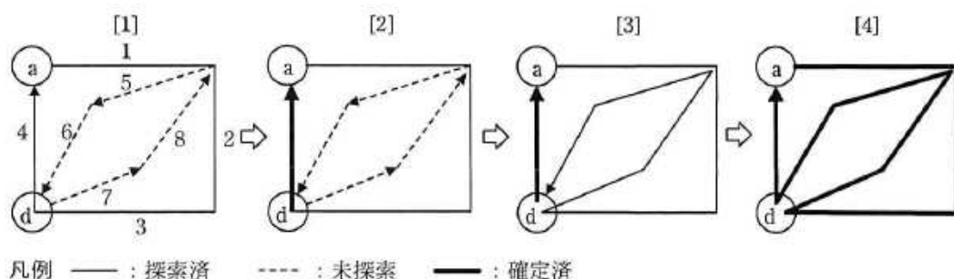
図 2 図 1 のグラフで点 a を出発点とした一筆書きの経路の求め方
