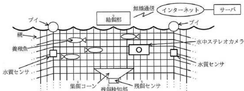
図 1 スマート生け簀 す の概観
