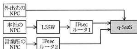
図 4 外出先及び社内の NPC から q-SaaS アクセス時に経由する社内の機器
