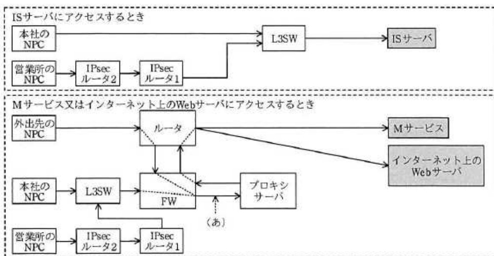
図 2 NPC による各種通信時に経路する社内の機器又はサーバ
